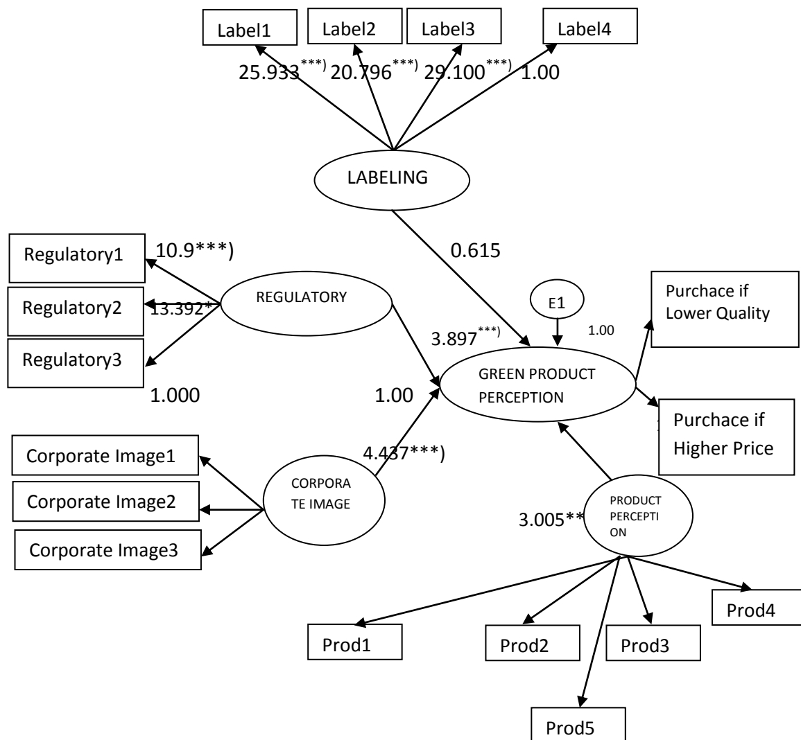
Gambar 2 Model Persamaan Struktural
